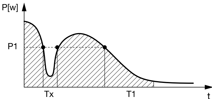
Kuva 69: Viivästyskäyrä tehon laskiessa / häiriötilanteessa
