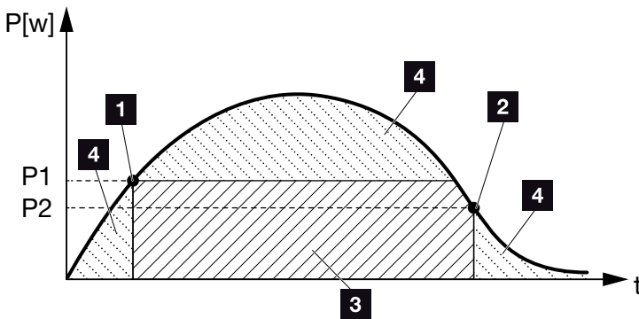
Kuva 67: Oman kulutuksen (toiminto 2) käyrä
